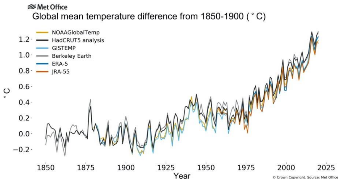
Figur 3 - Global middeltemperatur i perioden 1850 til 2020 set i forhold til, hvad temperaturen var før industrialiseringen (global middeltemperatur i perioden 1850 til 1900)
