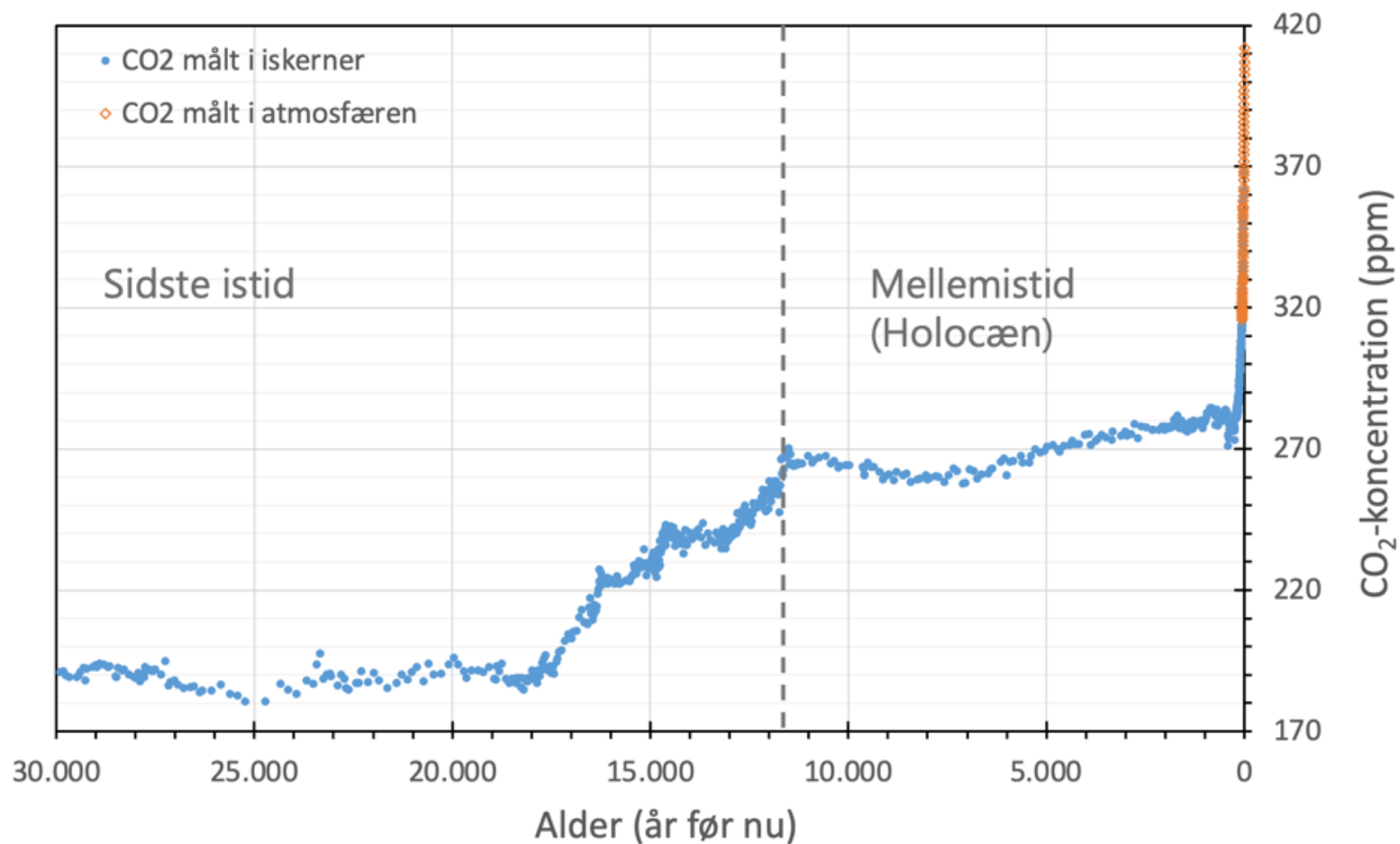
Figur 1 - Atmosfæriske CO 2 -koncentrationer gennem de sidste 800.000 år fra henholdsvis iskerner (blå) og målinger direkte i atmosfæren (orange). Her er der zoomet ind på de sidste 30.000 år for at kunne sammenligne den moderne stigning i CO 2 (helt til højre) med stigningen, da sidste istid sluttede (midt i figuren).
